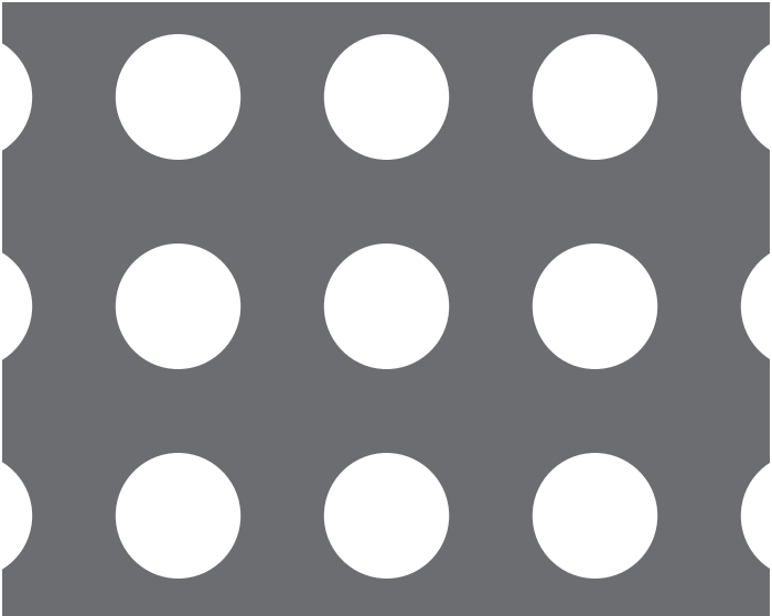
【No. 36】φ15-P25 並列 28.3%
