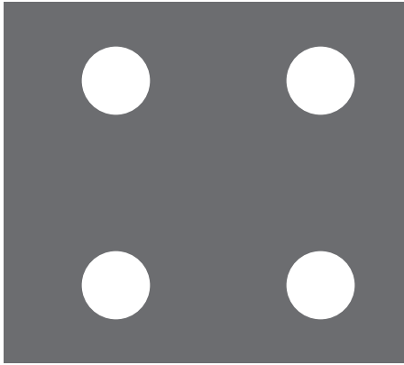
【No. 31】φ10-P30 並列 8.7%
