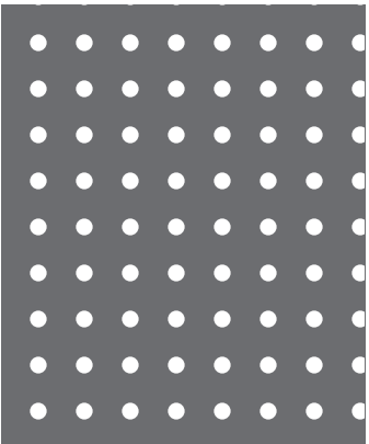
【No. 4】φ2-P5.5 並列 10.4%
