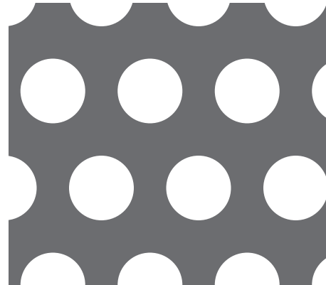
【No. 43】φ12-P18 60° 千鳥 40.2%
