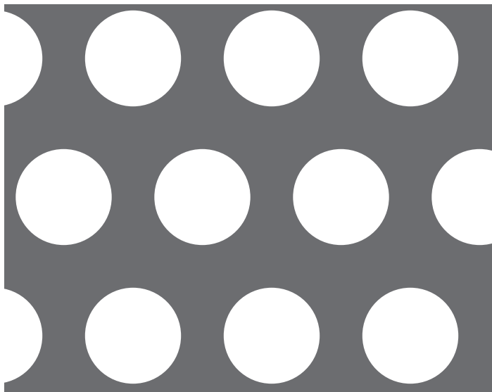
【No. 49】φ18-P26 60° 千鳥 43.4%
