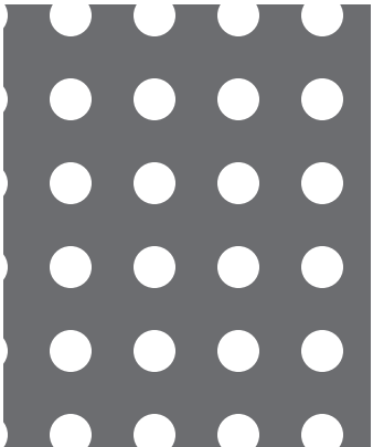
【No. 14】φ5-P10 並列 19.6%
