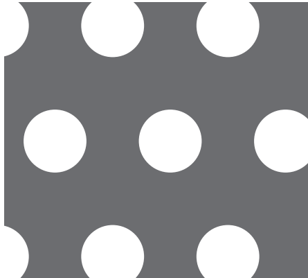
【No. 45】φ12-P22 60° 千鳥 27.0%
