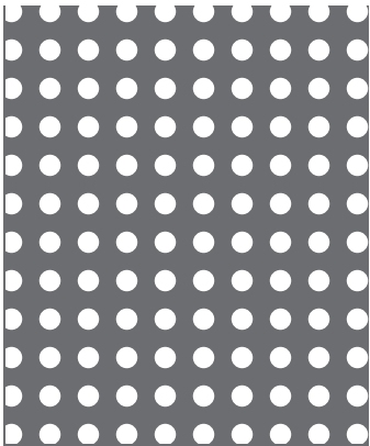
【No. 5】φ2.5-P4.5 並列 24.2%
