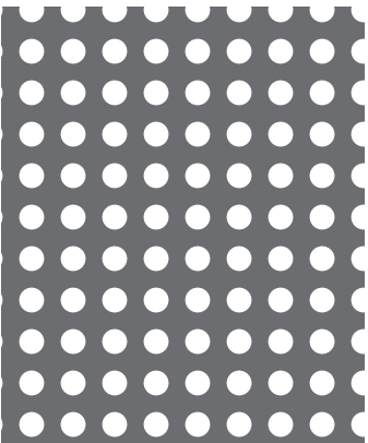
【No. 8】φ3-P5 並列 28.3%
