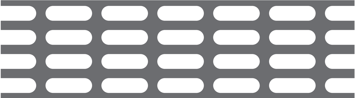
【No. 16】長孔 8×25-P13×30 47.8%
