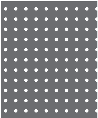
【No. 2】φ1.5-P4.5 並列 8.7%
