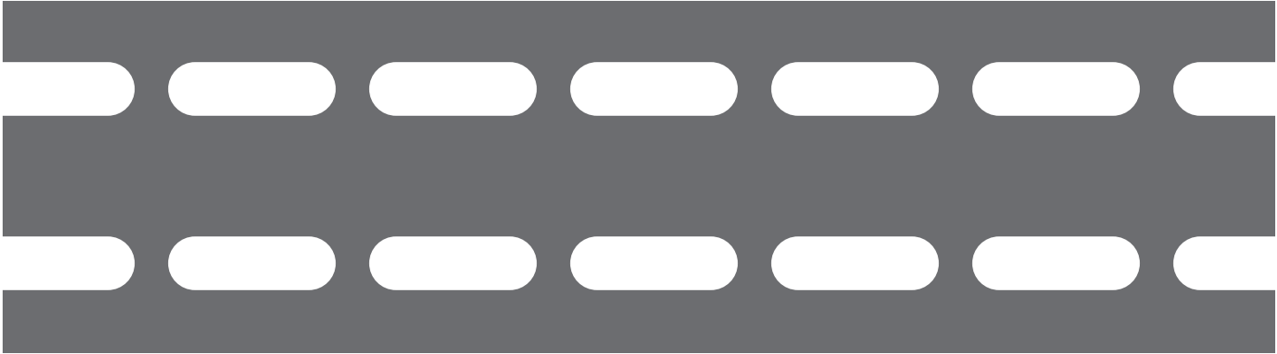
【No. 17】長孔 8×25-P26×30 23.9%
