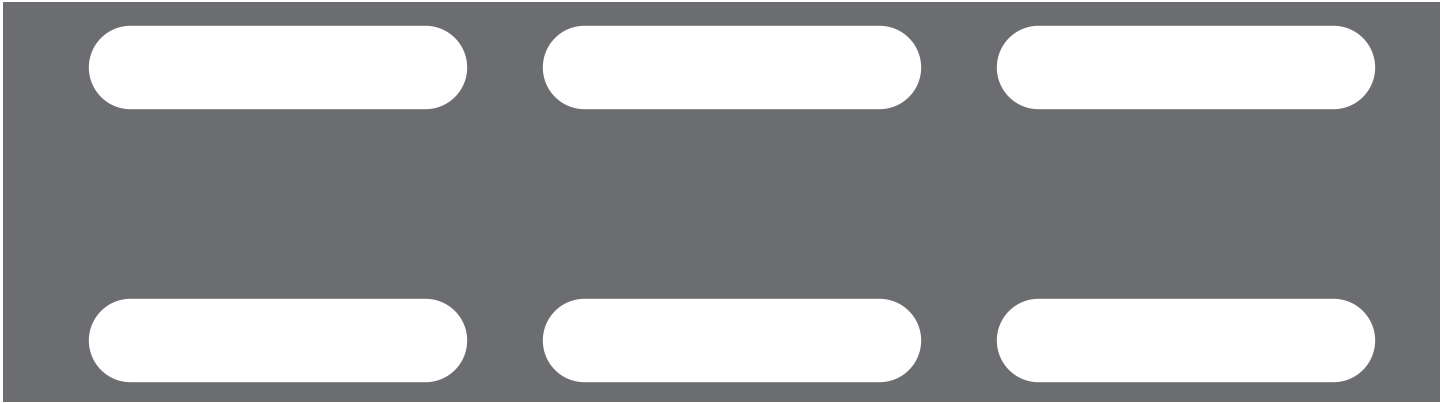
【No. 19】長孔 11×50-P36×60 24.3%
