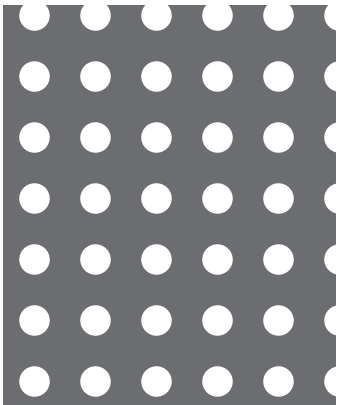
【No. 11】φ4-P8 並列 19.6%
