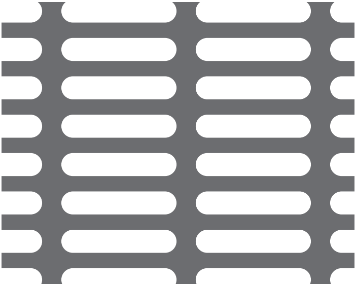
【No. 14】長孔 6×30-P10×35 49.2%
