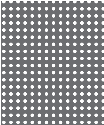
【No. 1】φ1.5-P3 並列 19.6%
