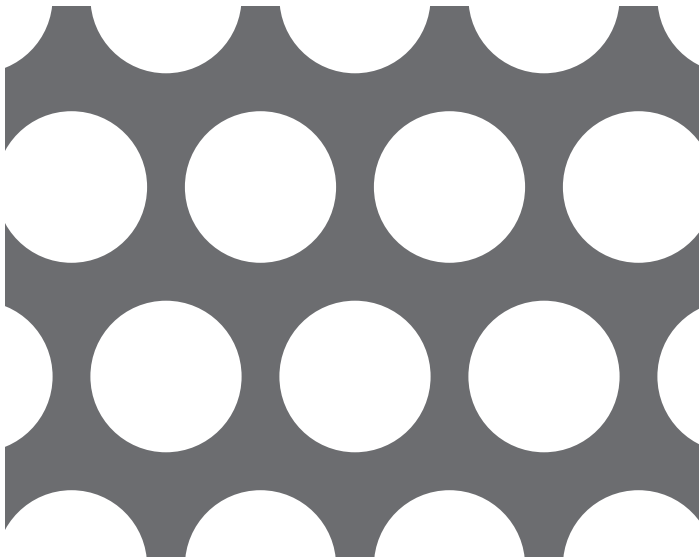
【No. 50】φ20-P25 60° 千鳥 57.9%
