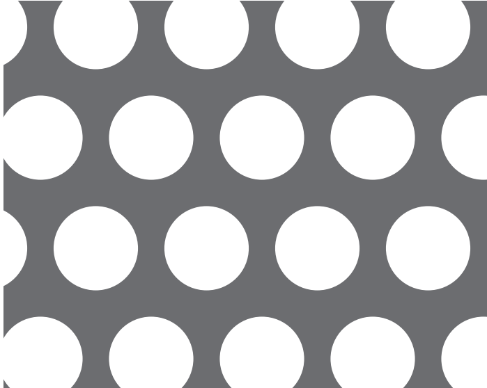
【No. 48】φ16-P21 60° 千鳥 52.6%
