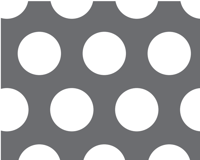
【No. 51】φ20-P30 60° 千鳥 40.2%
