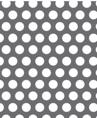
【No. 11】φ 4-P6 60° 千鳥 40.2%
