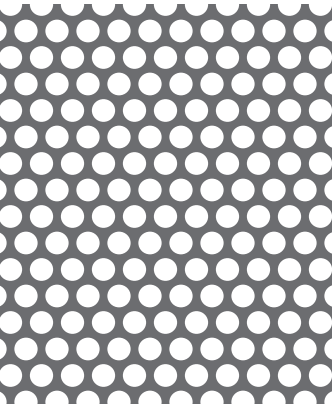
【No. 6】φ 3-P4 60° 千鳥 50.9%
