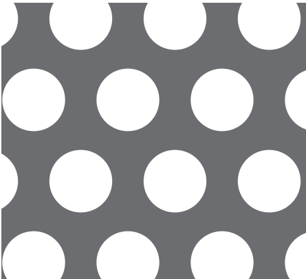
【No. 43】φ12-P18 60° 千鳥 40.2%
