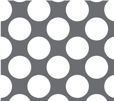
【No. 23】φ12-P20 45° 千鳥 56.5%
