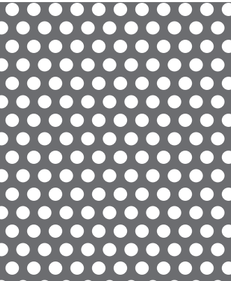
【No. 4】φ 2.5-P4 60° 千鳥 35.4%
