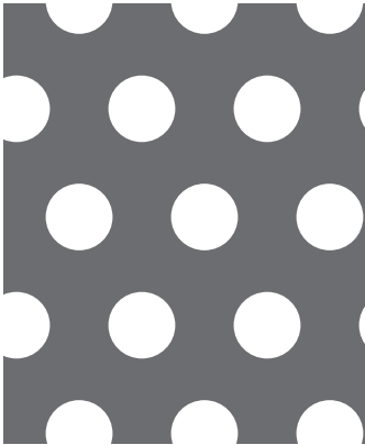
【No. 34】φ8-P15 60° 千鳥 25.7%
