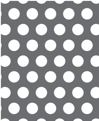
【No. 19】φ 5-P8 60° 千鳥 35.4%
