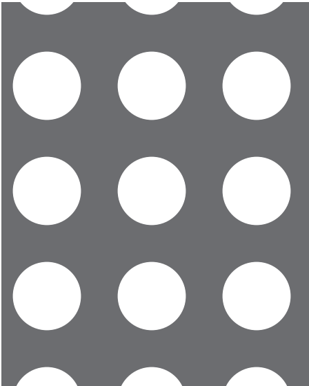
【No. 34】φ13-P20 並列 33.2%
