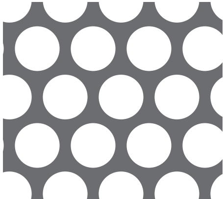
【No. 42】φ12-P15 60° 千鳥 57.9%
