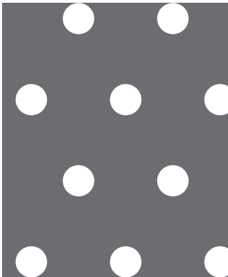
【No. 26】φ 6-P18 60° 千鳥 10.0%
