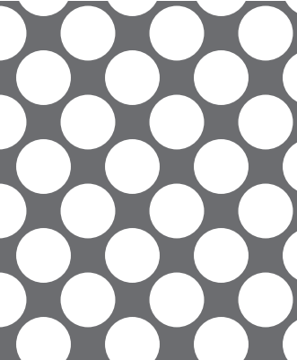
【No. 16】φ8-P13 45° 千鳥 59.5%
