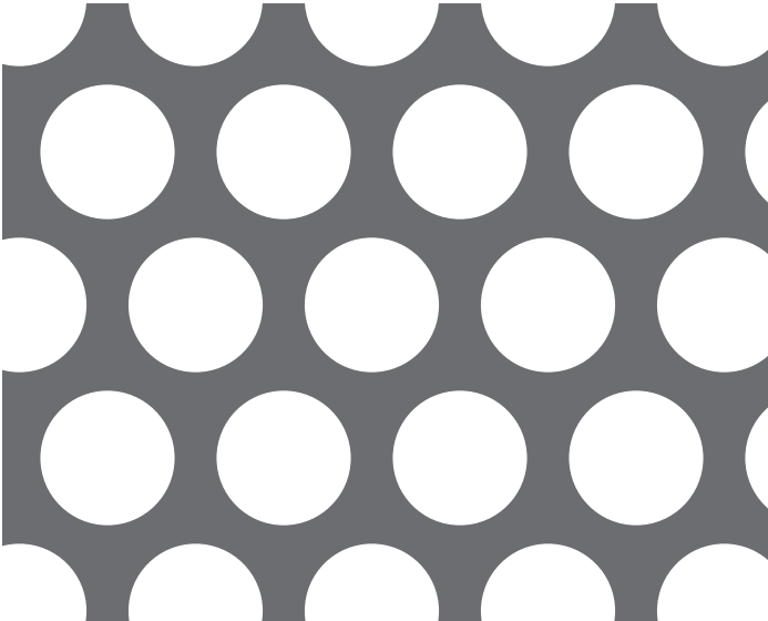
【No. 48】φ16-P21 60° 千鳥 52.6%
