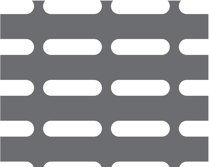
【No. 15】長丸孔 7×26-P18×30 31.8%
