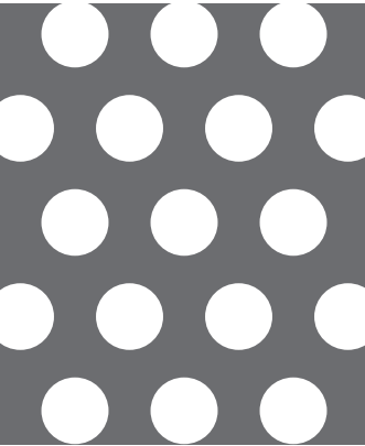
【No. 33】φ8-P13 60° 千鳥 34.3%
