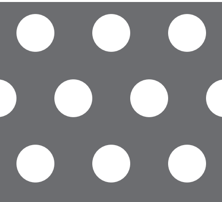
【No. 41】φ10-P20 60° 千鳥 22.6%
