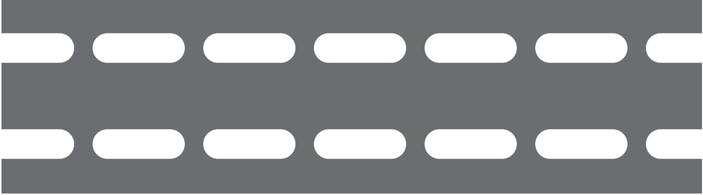
【No. 17】長丸孔 8×25-P26×30 23.9%
