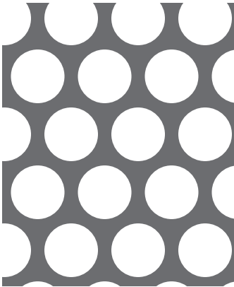
【No. 38】φ10-P12.5 60° 千鳥 57.9%
