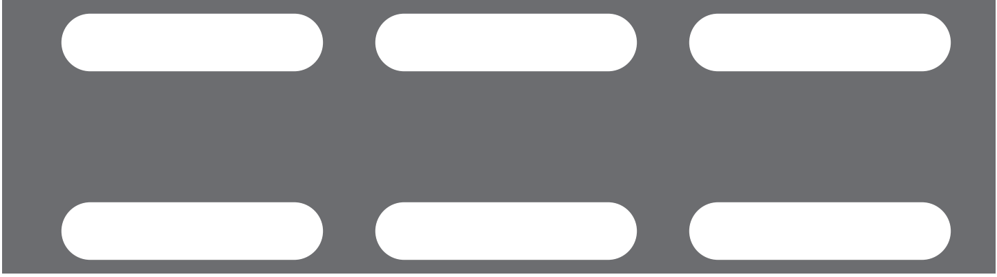
【No. 19】長丸孔 11×50-P36×60 24.3%
