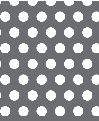
【No. 16】φ 4.5-P8 60° 千鳥 28.7%
