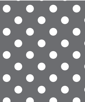
【No. 10】φ4-P12 45° 千鳥 17.4%
