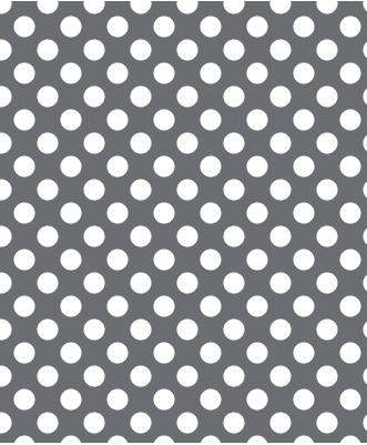
【No. 4】φ2.5-P5.5 45° 千鳥 32.4%
