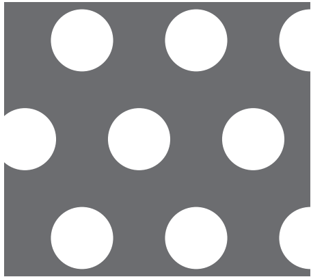
【No. 45】φ12-P22 60° 千鳥 27.0%
