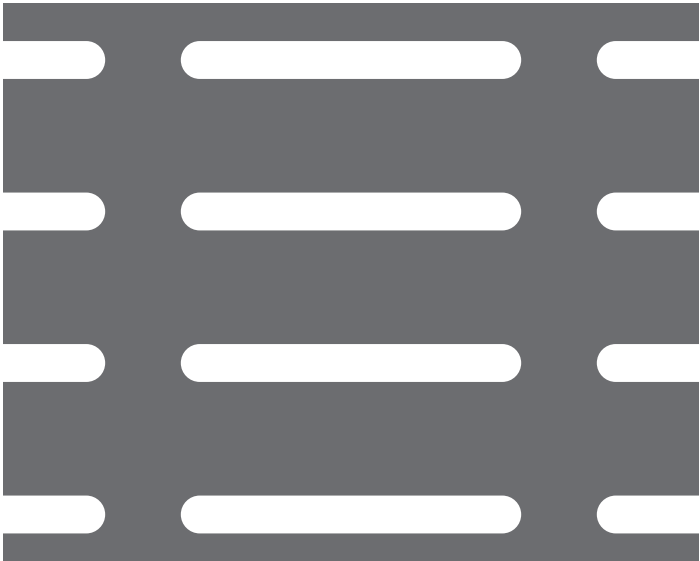
【No. 12】長丸孔 5×45-P20×55 20.0%
