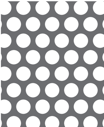
【No. 22】φ 6-P8 60° 千鳥 50.9%
