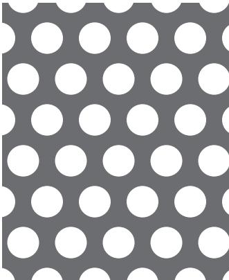
【No. 23】φ 6-P9 60° 千鳥 40.2%
