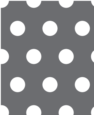
【No. 30】φ 7-P15 60° 千鳥 19.7%
