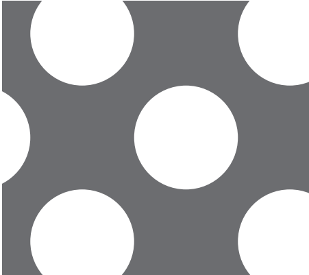
【No. 26】φ20-P40 45° 千鳥 39.3%
