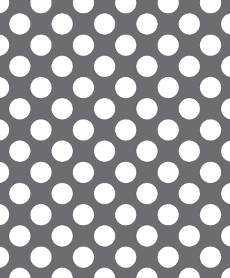
【No. 8】φ4-P8 45° 千鳥 39.3%
