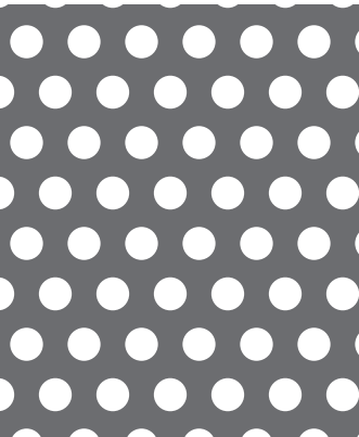
【No. 12】φ 4-P7 60° 千鳥 29.6%
