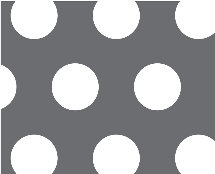
【No. 52】φ20-P35 60° 千鳥 29.6%
