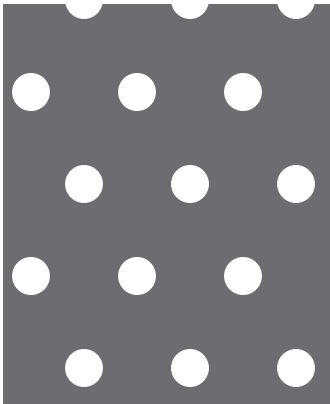
【No. 21】φ 5-P14 60° 千鳥 11.6%
