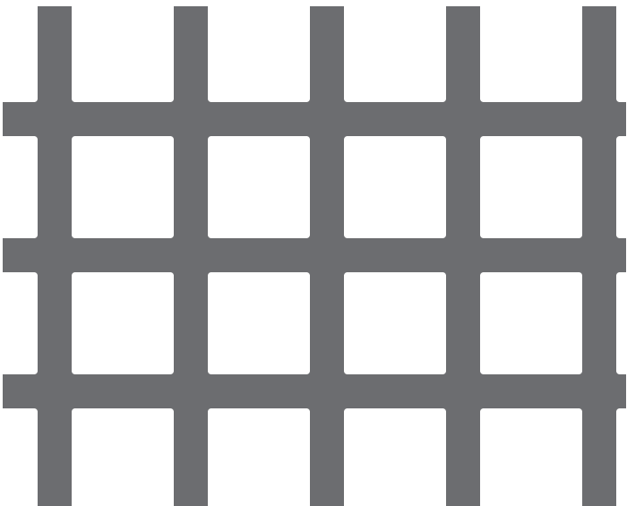
【No. 18】□15-P20 並列 56.3%
