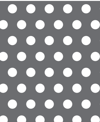
【No. 13】φ 4-P8 60° 千鳥 22.6%
