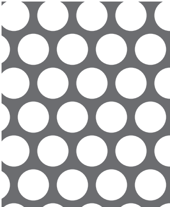
【No. 31】φ 8-P10 60° 千鳥 57.9%
