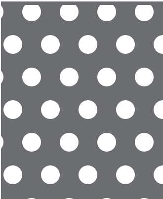
【No. 20】φ 5-P10 60° 千鳥 22.6%
