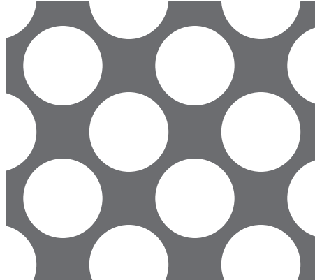
【No. 25】φ15-P25 45° 千鳥 56.5%
