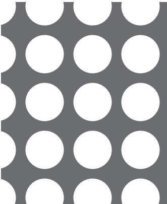
【No. 28】φ10-P12.5 並列 50.2%
