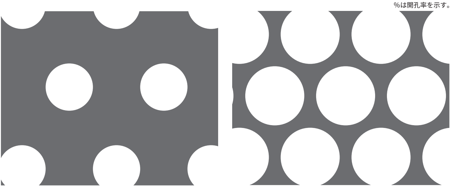
【No. 53】φ20-P40 60°千鳥 22.7%
