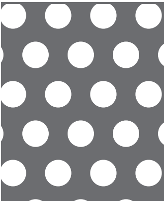
【No. 28】φ 7-P12 60° 千鳥 30.8%
