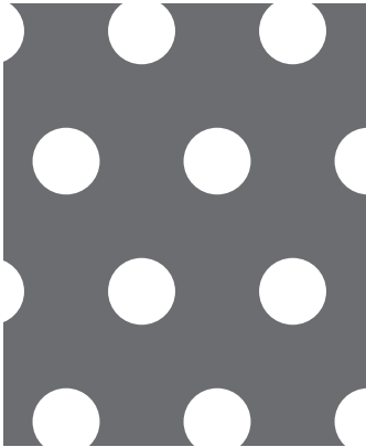
【No. 35】φ8-P18 60° 千鳥 17.9%
