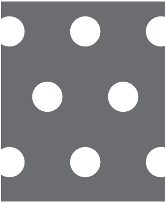
【No. 36】φ8-P20 60° 千鳥 14.5%
