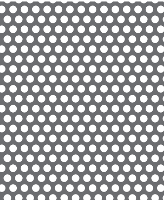
【No. 2】φ 2-P3 60° 千鳥 40.2%
