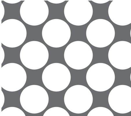
【No. 24】φ13-P20 45° 千鳥 66.3%
