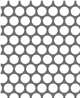
【No. 17】φ 5-P6 60° 千鳥 62.9%
