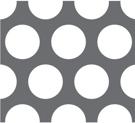
【No. 46】φ15-P20 60° 千鳥 50.9%
