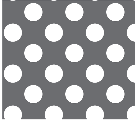
【No. 19】φ8-P18 45° 千鳥 31.0%
