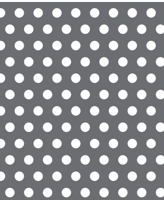
【No. 5】φ 2.5-P5 60° 千鳥 22.6%
