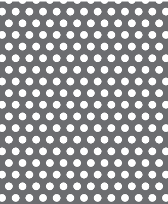
【No. 3】φ 2-P3.5 60° 千鳥 29.6%
