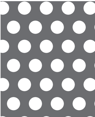
【No. 24】φ 6-P10 60° 千鳥 32.6%
