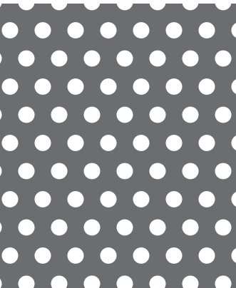
【No. 8】φ 3-P6 60° 千鳥 22.6%
