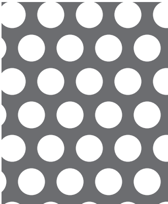
【No. 27】φ 7-P10 60° 千鳥 44.3%
