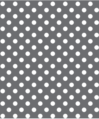
【No. 3】φ2-P5.5 45° 千鳥 20.8%
