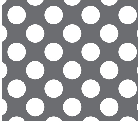
【No. 18】φ8-P16 45° 千鳥 39.3%
