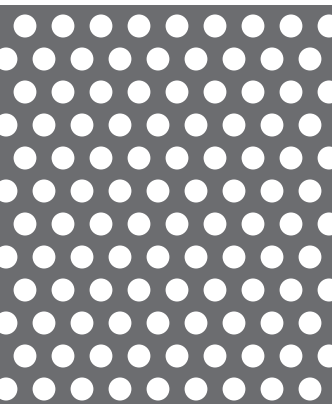
【No. 7】φ 3-P5 60° 千鳥 32.6%
