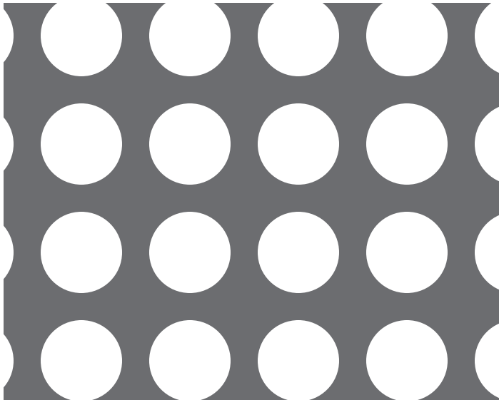
【No. 35】φ15-P20 並列 44.2%
