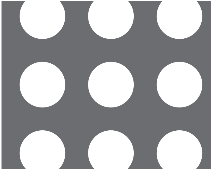
【No. 37】φ20-P30 並列 34.9%
