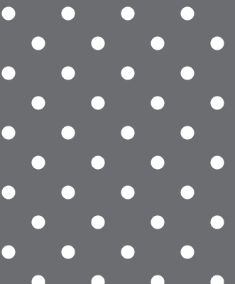
【No. 5】φ2.5-P11 45° 千鳥 8.1%
