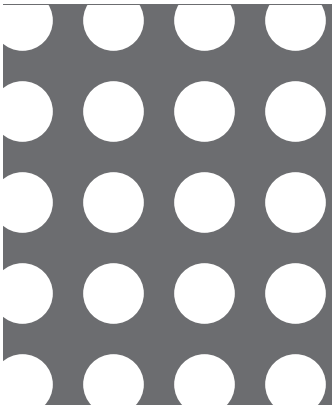
【No. 22】φ8-P12 並列 34.9%
