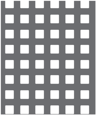
【No. 2】□4-P7 並列 32.7%
