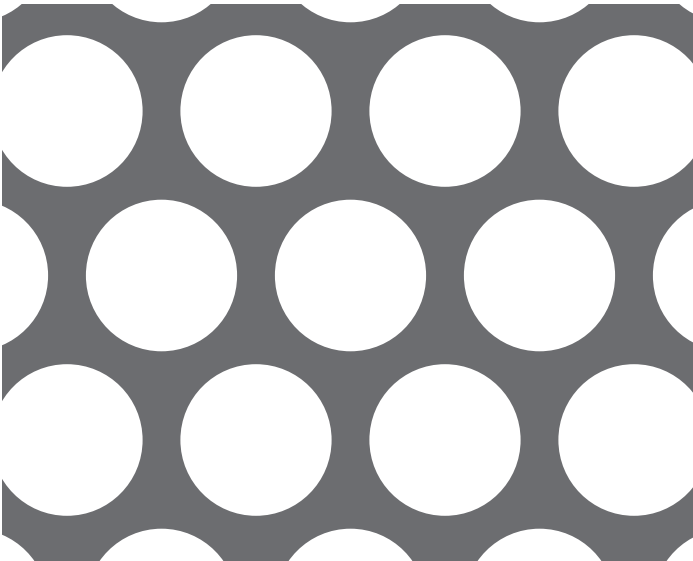
【No. 50】φ20-P25 60° 千鳥 57.9%
