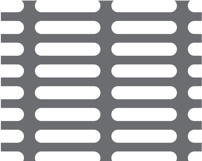
【No. 14】長丸孔 6×30-P10×35 49.2%
