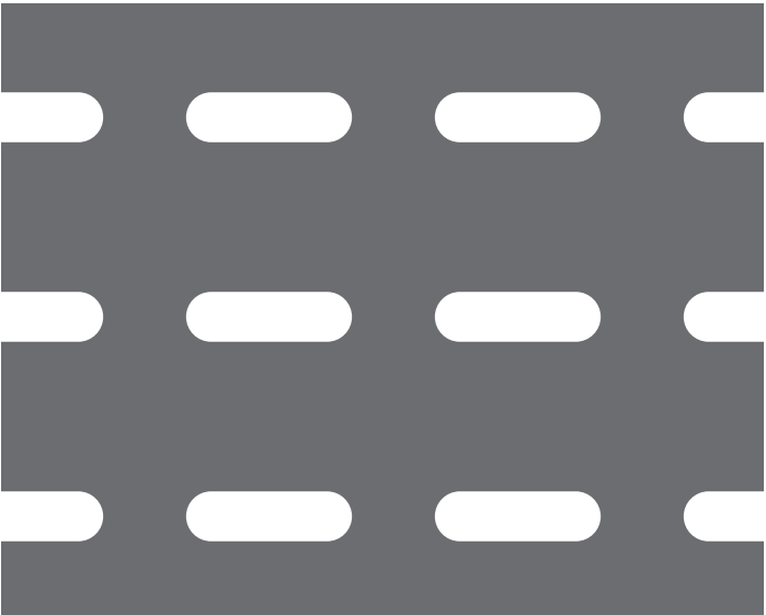
【No. 13】長丸孔 6×20-P24×30 15.6%
