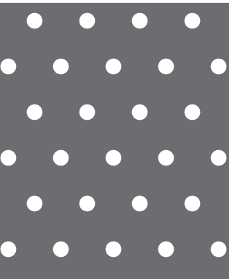
【No. 9】φ 3-P10 60° 千鳥 8.2%
