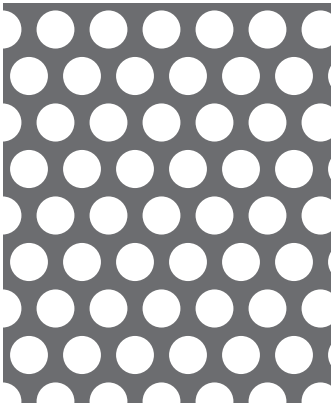
【No. 18】φ 5-P7 60° 千鳥 46.2%
