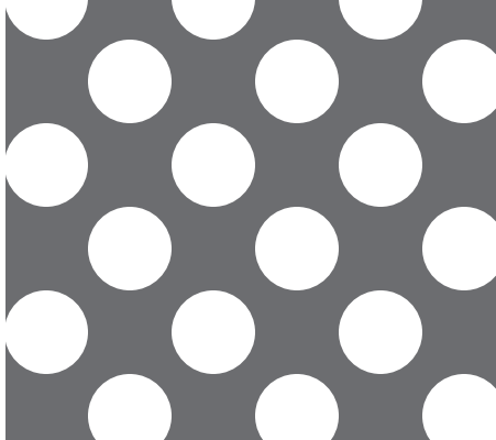
【No. 21】φ10-P20 45° 千鳥 39.2%
