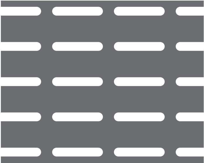
【No. 10】長丸孔 4×23-P16×28 19.8%
