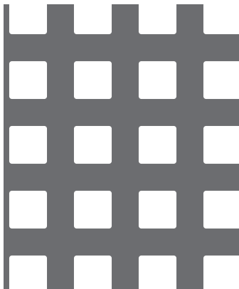
【No. 8】□7-P12 並列 34.0%
