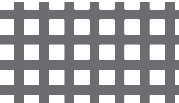
【No. 13】□8-P13 並列 37.9%
