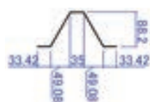
断面図
