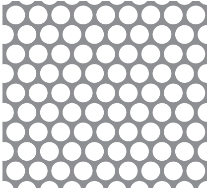
05-06 φ5-P6 60° 千鳥 62.9%
