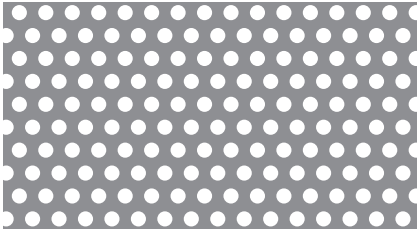
02-035 φ2-P3.5 60° 千鳥 29.6%
