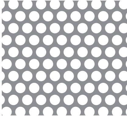
045-06 φ4.5-P6 60° 千鳥 50.9%
