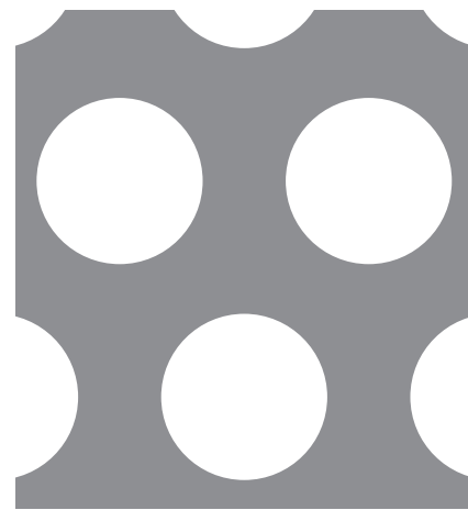
20-30 φ20-P30 60° 千鳥 40.2%
