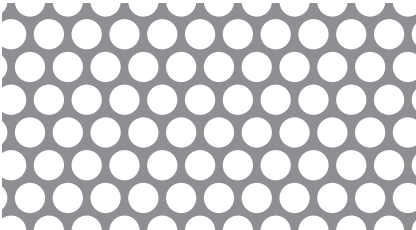
04-05 φ4-P5 60° 千鳥 57.9%
