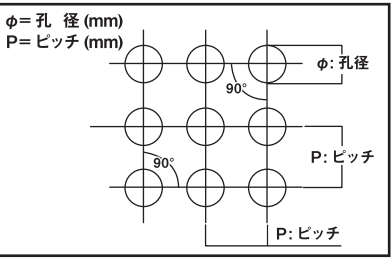
丸孔並列
