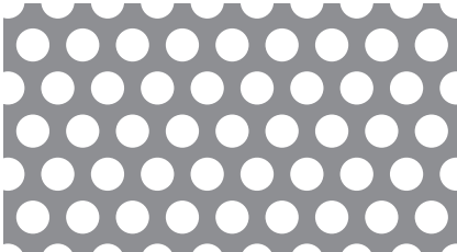
04-06 φ4-P6 60° 千鳥 40.2%
