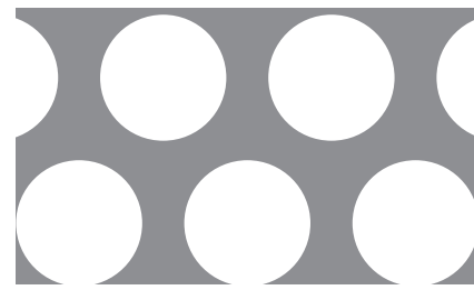
15-20 φ15-P20 60° 千鳥 50.9%
