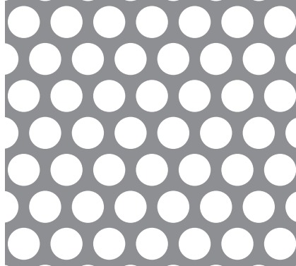
06-08 φ6-P8 60° 千鳥 50.9%
