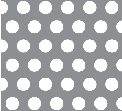
06-10 φ6-P10 60° 千鳥 32.6%
