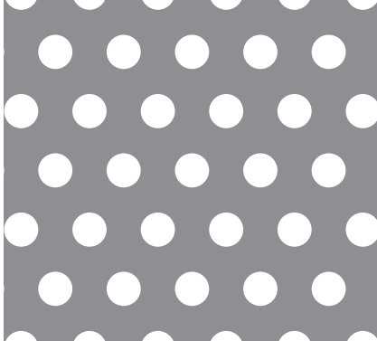
05-10 φ5-P10 60° 千鳥 22.6%
