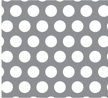
06-09 φ6-P9 60° 千鳥 40.2%
