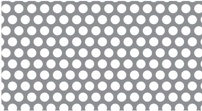
025-035 φ2.5-P3.5 60° 千鳥 46.2%
