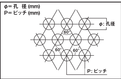
丸孔 60° 千鳥
