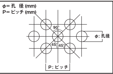
丸孔 45° 千鳥
