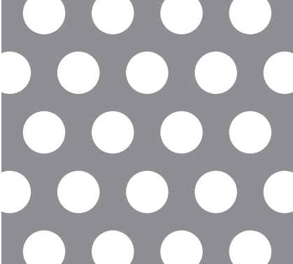
08-13 φ8-P13 60° 千鳥 34.3%
