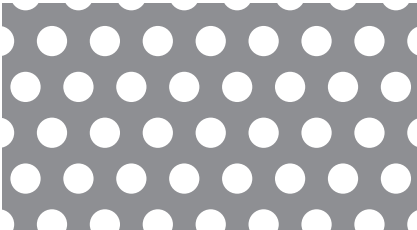
04-07 φ4-P7 60° 千鳥 29.6%
