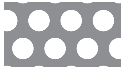
10-15 φ10-P15 60° 千鳥 40.2%
