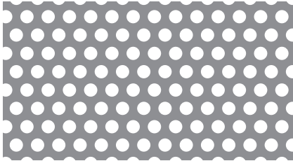
025-04 φ2.5-P4 60° 千鳥 35.4%
