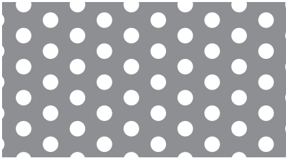
03-06 ※ φ3-P6 60° 千鳥 22.6%
