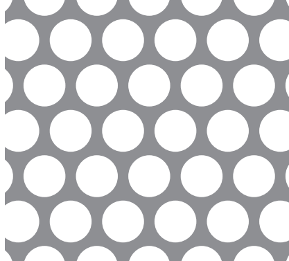
08-10 φ8-P10 60° 千鳥 57.9%
