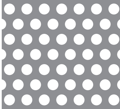
05-08 φ5-P8 60° 千鳥 35.4%
