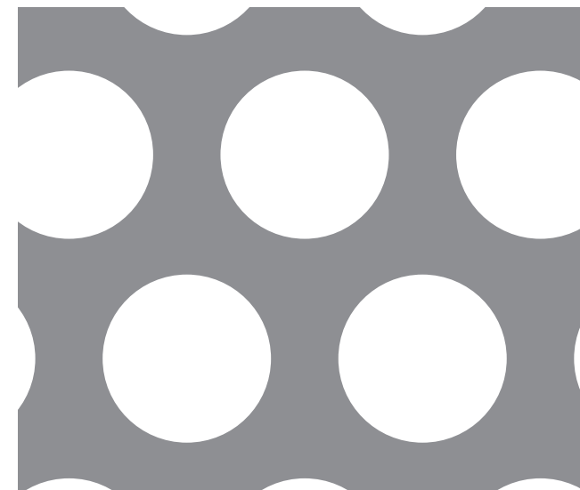
25-35 φ25-P35 60° 千鳥 46.2%
