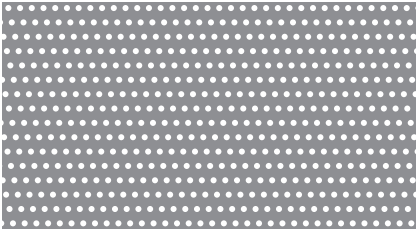
008-0155 φ0.8-P1.55 60° 千鳥 24.1%
