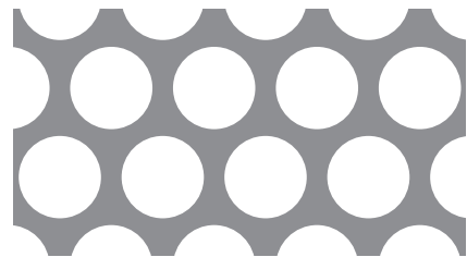
10-125 φ10-P12.5 60° 千鳥 57.9%
